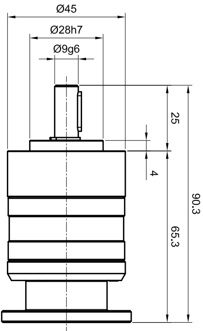
2 STAGES RATIO: 16:1 - 24:1 - 36:1
