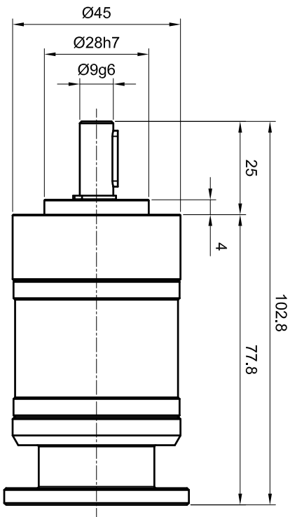
3 STAGES RATIO: 64:1 - 96:1 - 144:1 - 216:1
