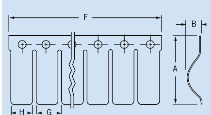
Door Finger 2801
