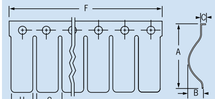
Door Finger 2802
