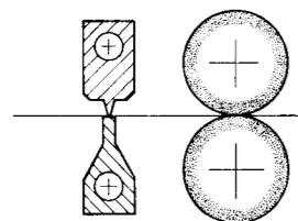
SALDATURA LATERALE RINFORZATA (BARRA CALDA) HEAVY DUTY SIDE SEAL SELLADO LATERAL CON REFUERZO
