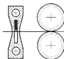
NASTRO DOPPIO DOUBLE BOTTOM SEAL SELLADO DE FONDO DOBLE
