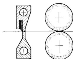
NASTRO SEMPLICE BOTTOM SEAL SELLADO DE FONDO SIMPLE
