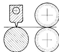
SALDATURA LATERALE (BARRA CALDA) SIDE SEAL SELLADO LATERAL
