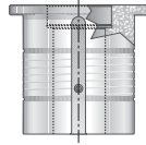
3-1/2" à 1-1/4" Adaptateur de guide de poinçon de station D LVD à station B tourelle épaisse LPLK00AD
