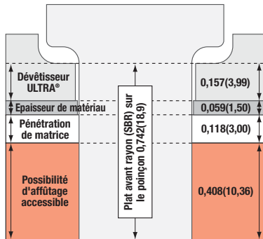
Système Mate ULTRA® avec poinçon ULTRA®
