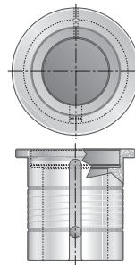
Adaptateur de guide de poinçon station 3-1/2" à 2" D à C APLJ00AD
