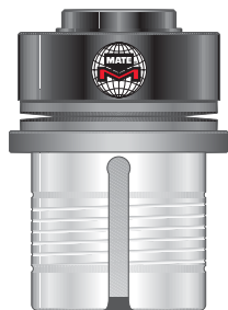
Guide ULTRA TEC® fully guided à dégagement de pinces
