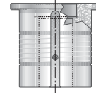
3-1/2" à 2" Adaptateur de guide de poinçon de station D LVD à station C tourelle épaisse LPLJ00AD
