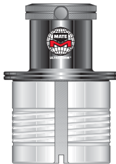
Guide de formage ULTRAFORM® type LVD LFKD2
