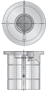
Adaptateur de guide de poinçon station 4-1/2" à 1-1/4" E à B APLM00AD
