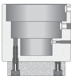
Support de serrage ULTRA® / Tourelle épaisse Ensemble avec entraînement 3/8" clé hexagonale 10 mm 2" Stations C, 3-1/2" D et 4-1/2" E MATE00083
