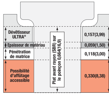
Système Mate ULTRA® avec poinçon type d'origine
