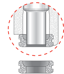
Dévêtisseur ULTRA® avec dégagement 0,118(3,0)
