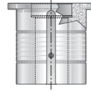
3-1/2" à 2" Adaptateur de guide de poinçon de station D LVD à station C LVD LPPJ00AD
