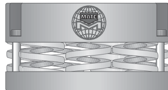
Ensemble ressorts Ultra Light™ (Jeu de 9) MATE00033 Ressorts rouge pression moyennement forte* MATE00281
