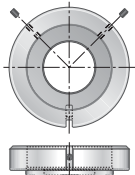
Adaptateur de matrice station 3-1/2" à 2" D à C* ADLJ00AD
