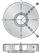
Adaptateur de matrice station 3-1/2" to 1-1/4" D à B* ADLK00AD
