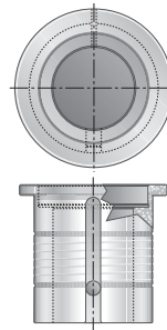
Adaptateur de guide de poinçon station 4-1/2" à 2" E à C APLL00AD
