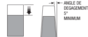
VUE DE HAUT ; AVEC ET SANS ANGLE DE DEGAGEMENT, MONTRANT L'EFFET DU DEPLACEMENT DU BORD AVANT DE LA LANGUETTE DANS LA MATRICE;
