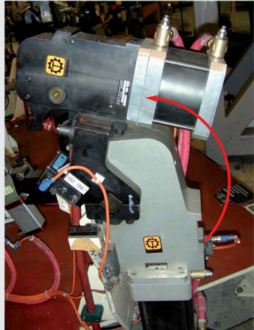
Einschwenken einer Lochzange PFS 200
