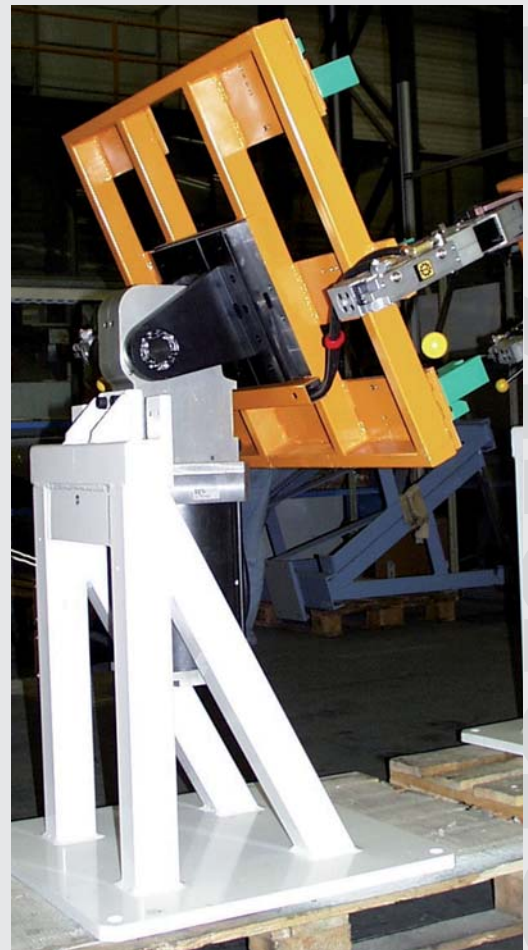
Antrieb für Schwenkeinheit als Kiptisch
