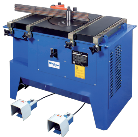
Special 42 S: schnelle, leistungsstarke Produktionsmaschine für Baustellen und für Biegebetriebe, mit robuster Stiftsteuerung. // Special 42 S: machine rapide et efficace pour chantiers et usines de cintrage, avec commande électromécanique à broches solide.
