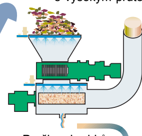
Pračka shrabků
