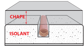
Insertion des gaines dans l'isolant
