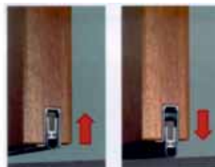
SEUIL MÉCANIQUE SOULEVABLE INTÉGRÉ AU VANTAIL
