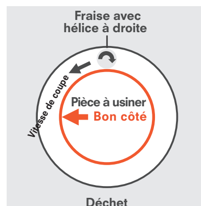
Forme découpée = pièce à usiner, vitesse de coupe dans le sens contraire des aiguilles d'une montre
