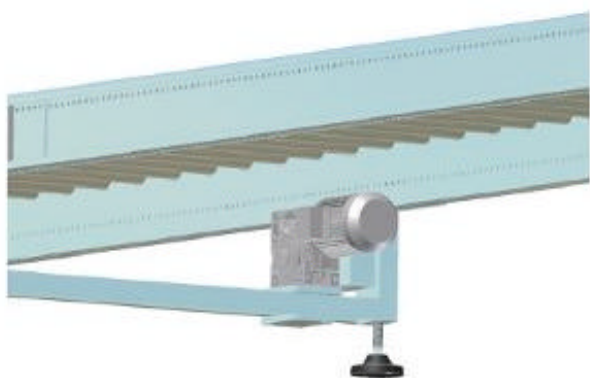
Motorizzazione con riduttore a vite senza fine
