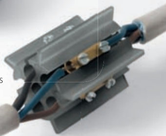
Jonction des câbles
