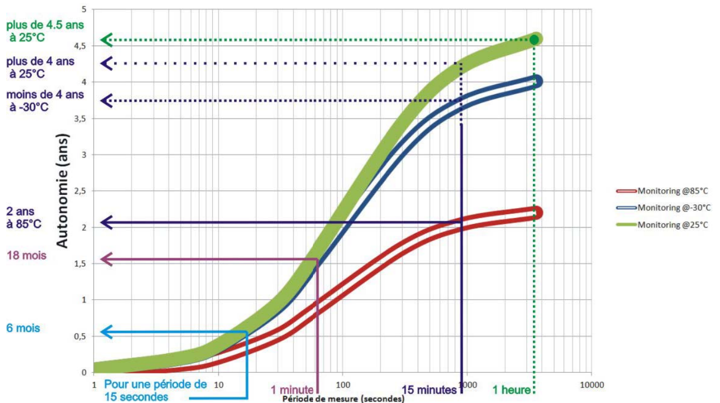
Newsteo LGR - Autonomie vs. Période de transmission
