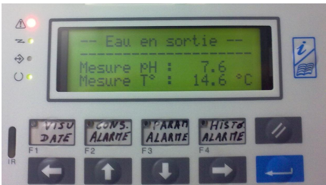
Détail de la console opérateur
