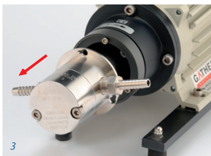
Retirer la tête de la pompe
