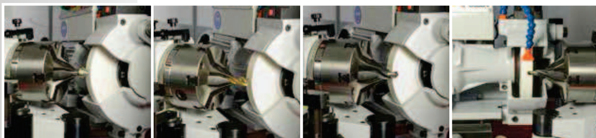
APE 40 UP - APE 40 AUTOMATIQUE - APE 60 EXEMPLES D'AFFÛTAGES
