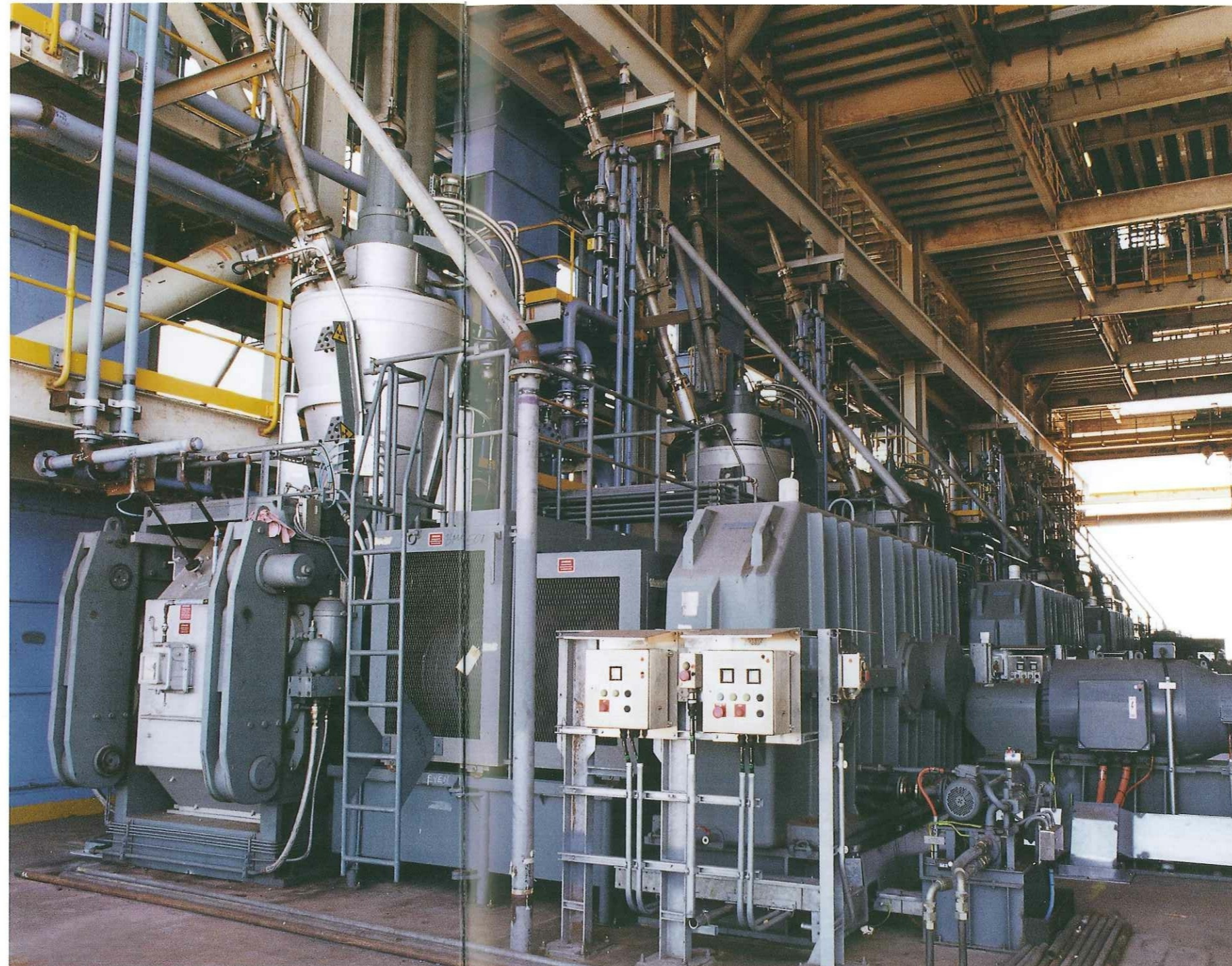
Briquetting machines for DRI-fines Brikettiermaschinen für DRI-Fines
