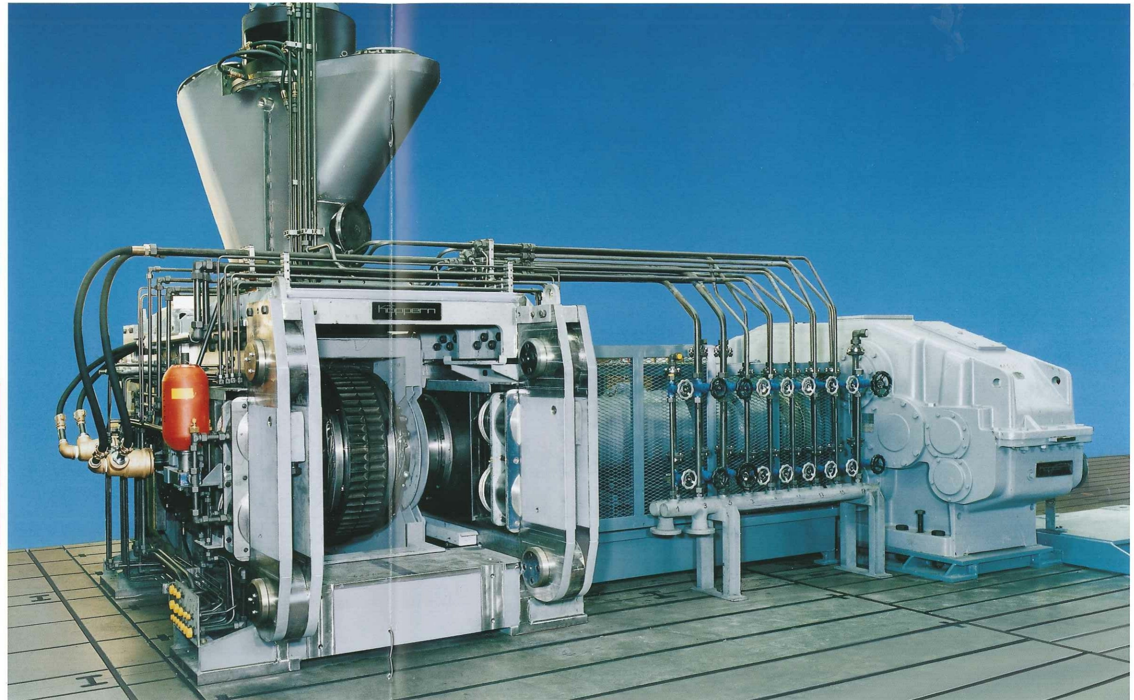
Köppern Roller Press for hot briquetting at 700° C Köppern-Walzenpresse für die Heissbrikettierung bei 700° C
