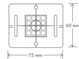
Plaquettes de mesure RS50/51 avec point de visée réflecteur 30 x 30 mm
