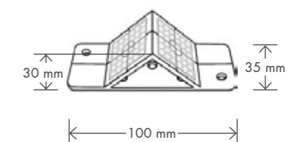
RSAK130 avec point de visée réflecteur 30 x 30 mm
