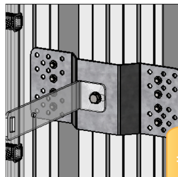
Paire de plaques de fixations sur bac acier (+ vis) Réf : 0733404
