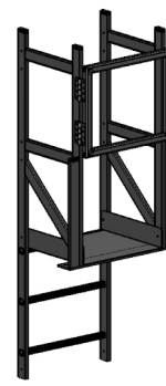
Kit Marche palière de 500 mm avec portillon de 500 mm assemblé - Réf : 0733504
