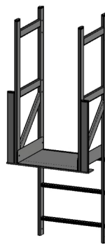
Kit marche palière de 500 mm - Réf : 0733503
