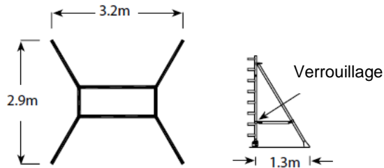
Dimensions avec petits stabilisateurs
