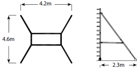
Dimensions avec grands stabilisateurs
