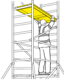
Mise en place du plancher par une seule personne
