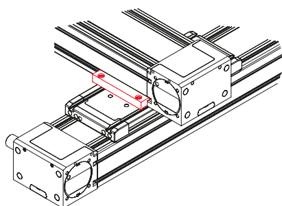
Fig. 2 : unités croisées
