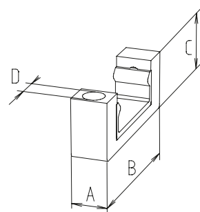
Pour interrupteur de fin de course
