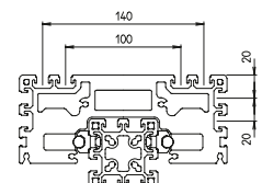
Profilé F-60
