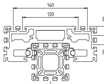
Profilé F-80
