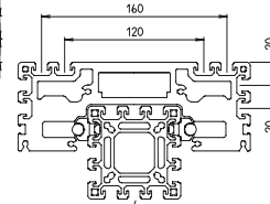
Profilé F-80
