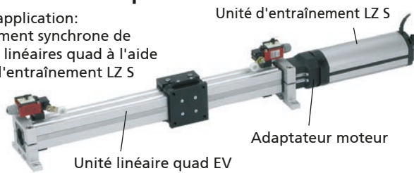
Autres adaptateurs disponibles sur demande
