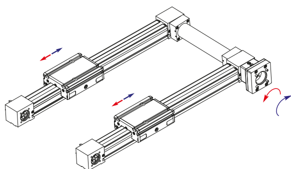
III. arbre synchronisé avec protection
