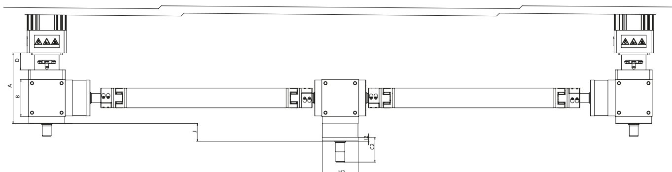
III. arbre Renvoi d'angle sur RK DuoLine S
