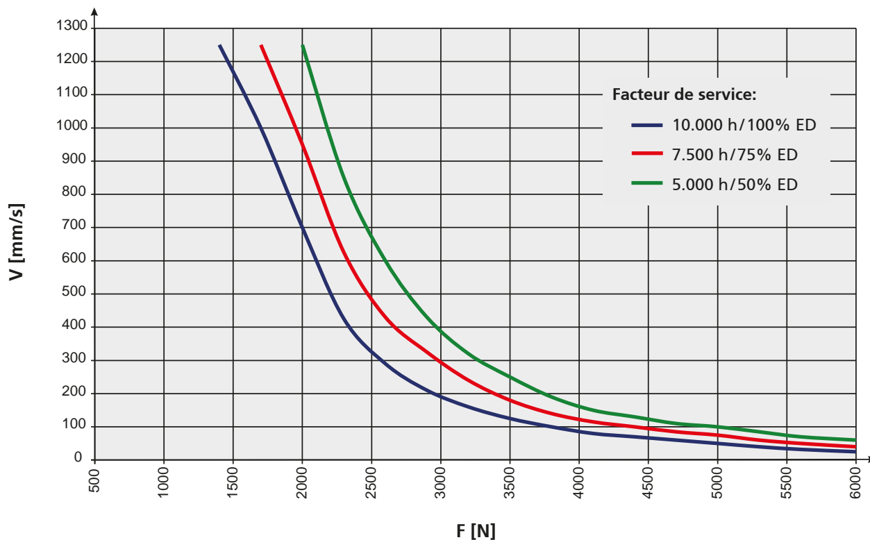
Diagramme vitesse / force SLZ 63 KG PL (KG 25x25) Pour courses > 700 mm, voir vitesse critique de la vis
