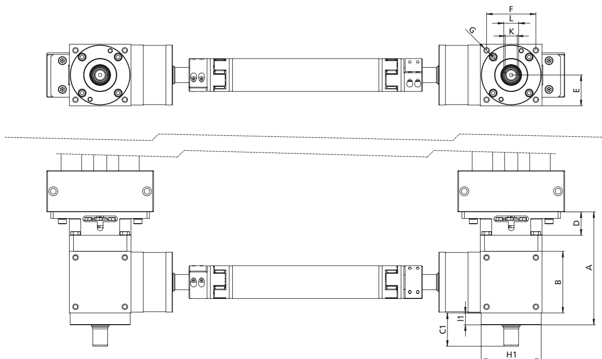
III. arbre Renvoi d'angle sur EPX-II KG
