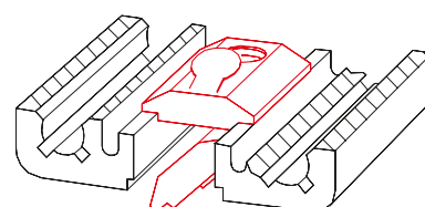
Écrou -K- à faire pivoter dans la rainure
