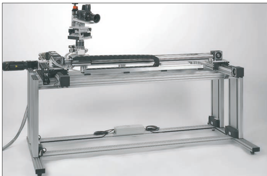
Réglage synchrone de 4 colonnes
