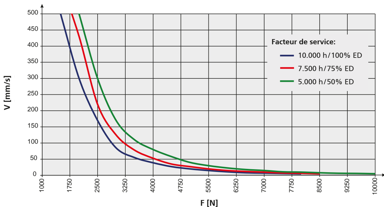
Diagramme vitesse / force SLZ 63 KG PL (KG 25x10) Pour courses > 700 mm, voir vitesse critique de la vis
