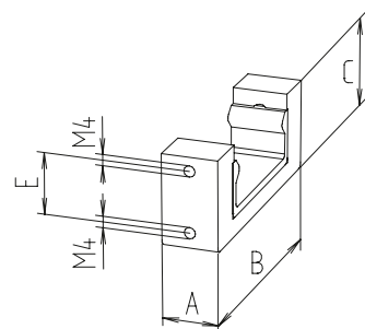
Pour interrupteur de fin de course
