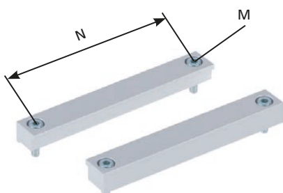
Modèle avec lamage
