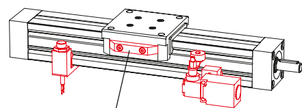
Clavette pour interrupteur de fin de course uniquement sur EV30 et 50 avec chariot de guidage fermé
