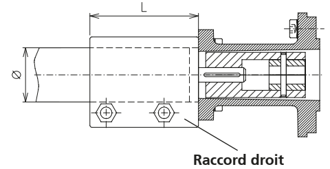
Uniquement pour les unités linéaires de type E
