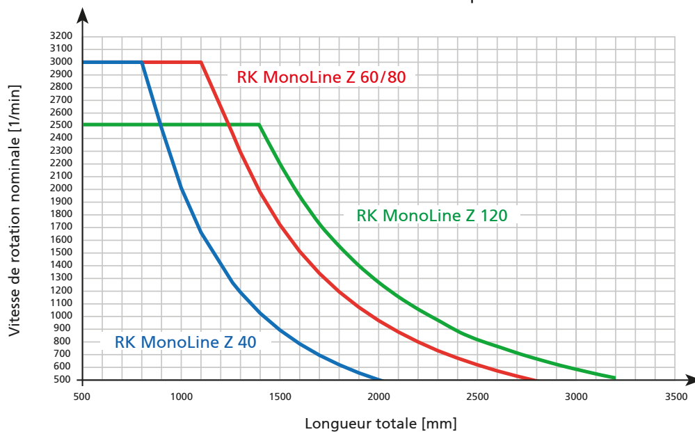
Vitesse de rotation critique
