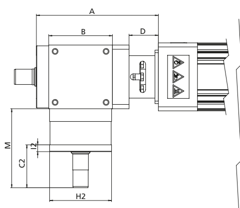
III. arbre Renvoi d'angle sur RK DuoLine S
