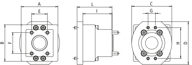
Autres adaptateurs disponibles sur demande
