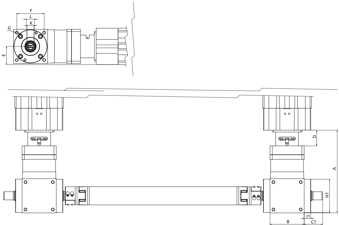
III. arbre Renvoi d'angle sur PLS
