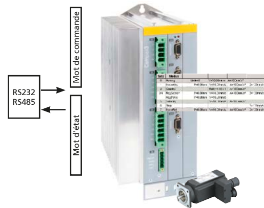
via RS232/RS485 à l'aide des mots de commande et d'état
