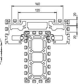
Profilé F-80 x 160
