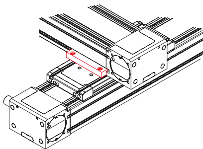
III. 2 : unités croisées
