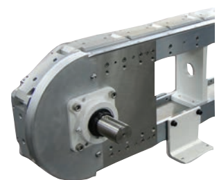
Takt-Palettenband- förderer
