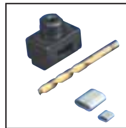
Outil à sertir et percer les tresses
